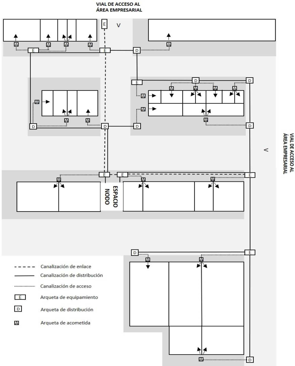
Figura 1. Esquema tipo de infraestructura de soporte de red de telecomunicaciones en un área empresarial
